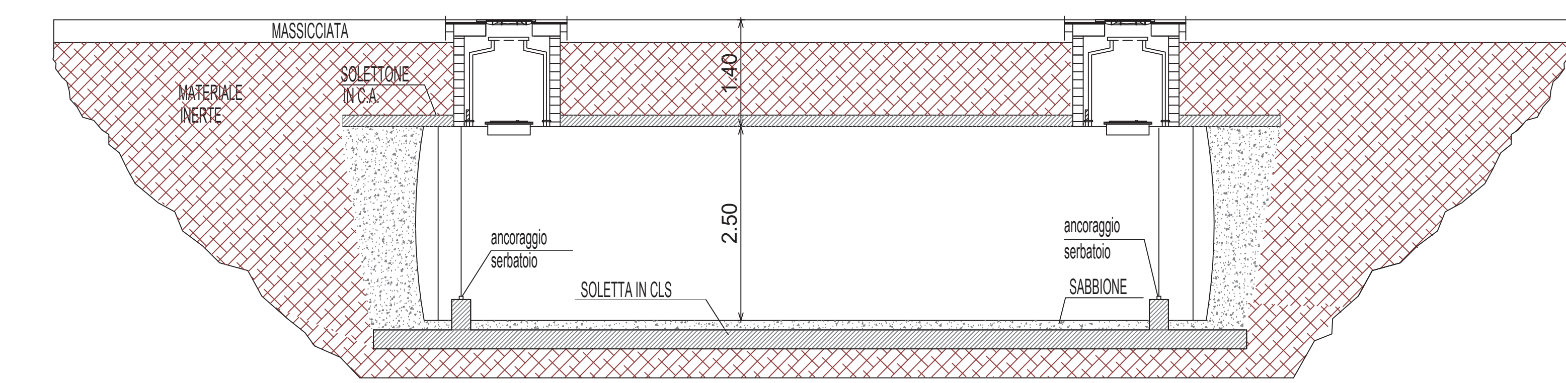
SEZIONE LATERALE SERBATOI
