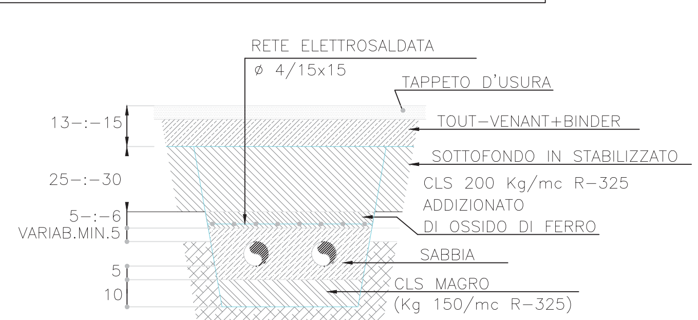
SEZIONE CUNICOLO IMPIANTO MECCANICO SU PAVIMENTAZIONI BITUMINOSE
