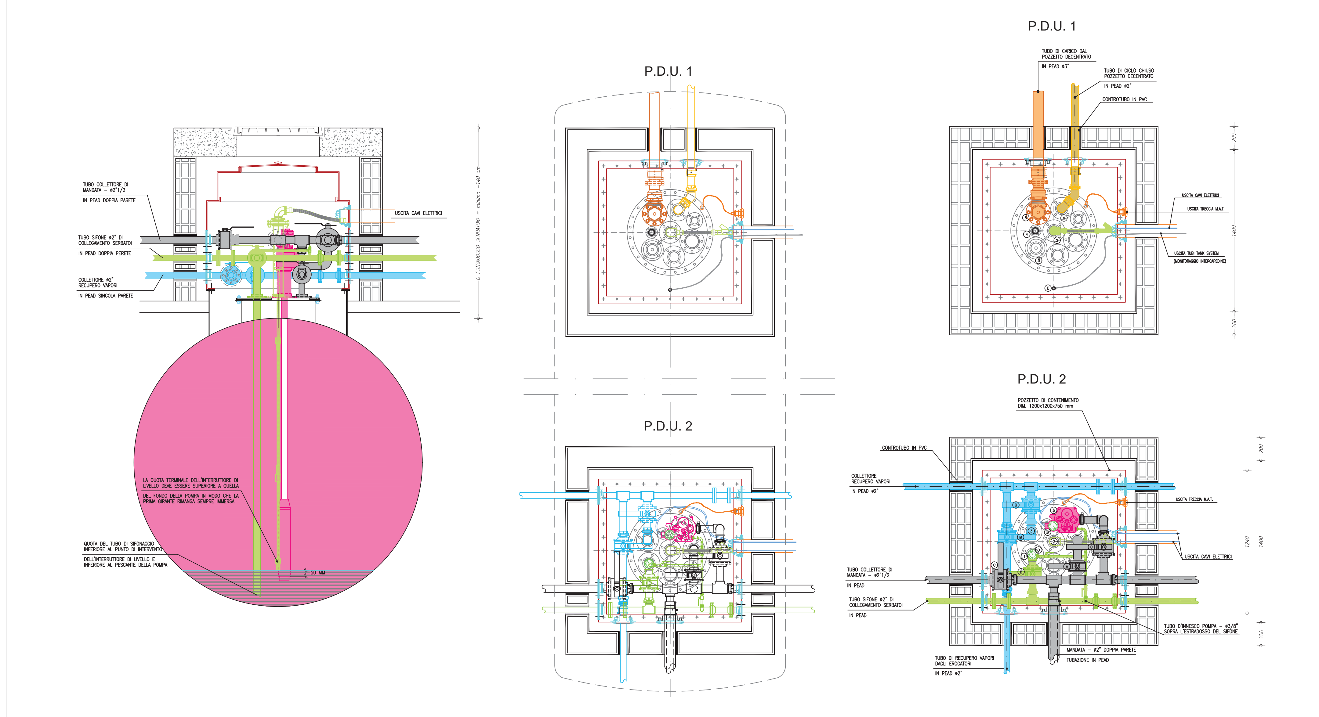
SEZIONE FRONTALE SERBATOI
