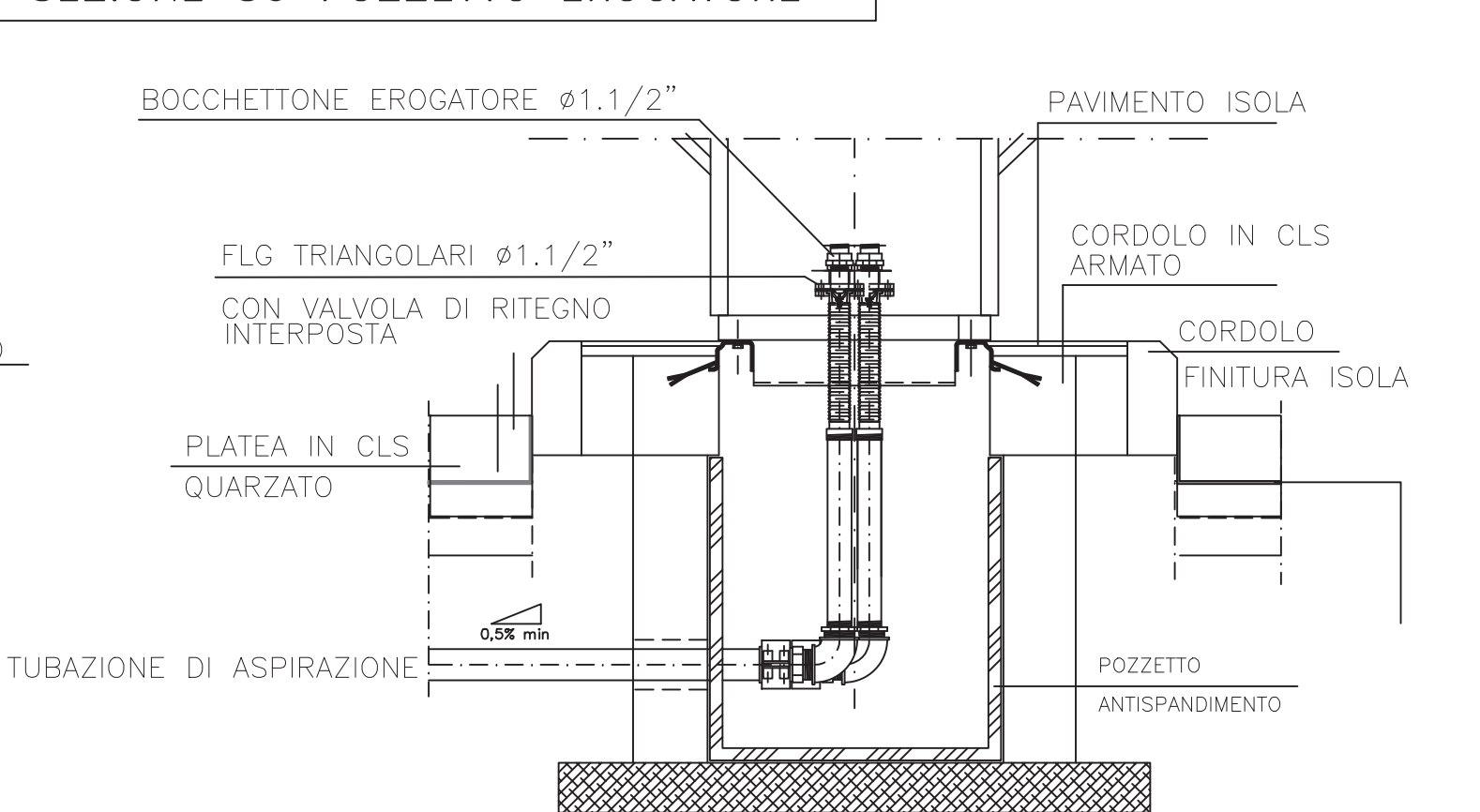
SEZIONE SU POZZETTO EROGATORE
