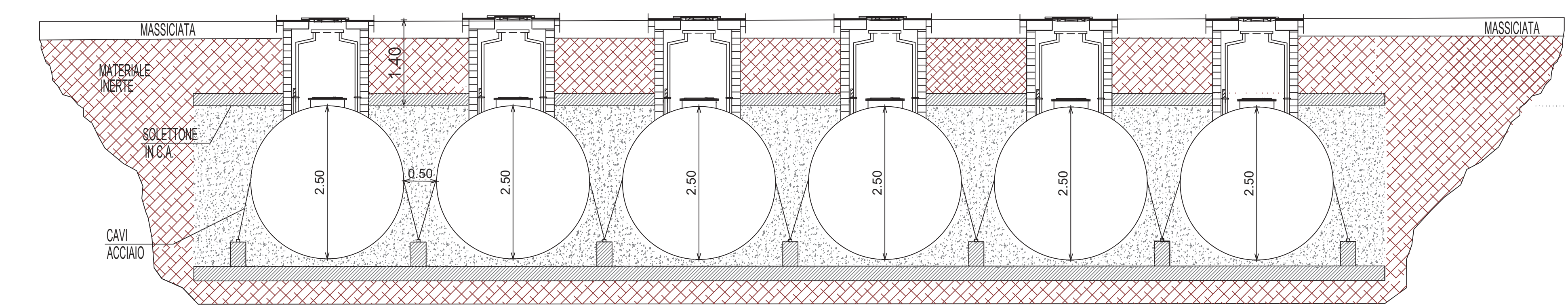
SEZIONE FRONTALE SERBATOI
