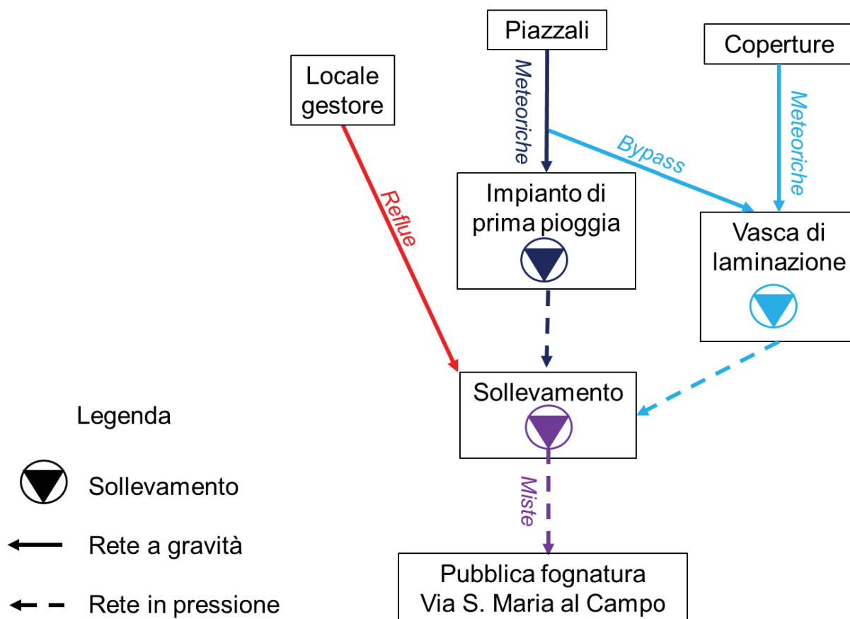
Figura 4 – Schematizzazione dell'impianto fognario
